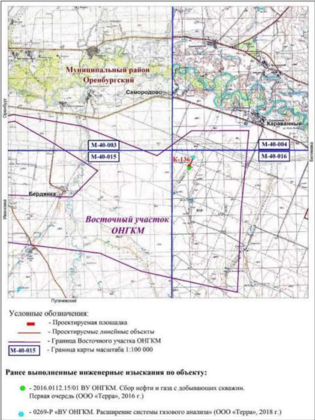
Рисунок 1 - Обзорная схема размещения объекта, совмещенная с топографо-геодезической изученностью
